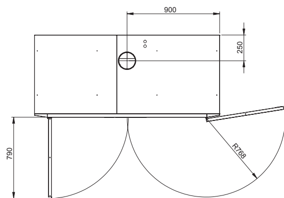
顶视图
